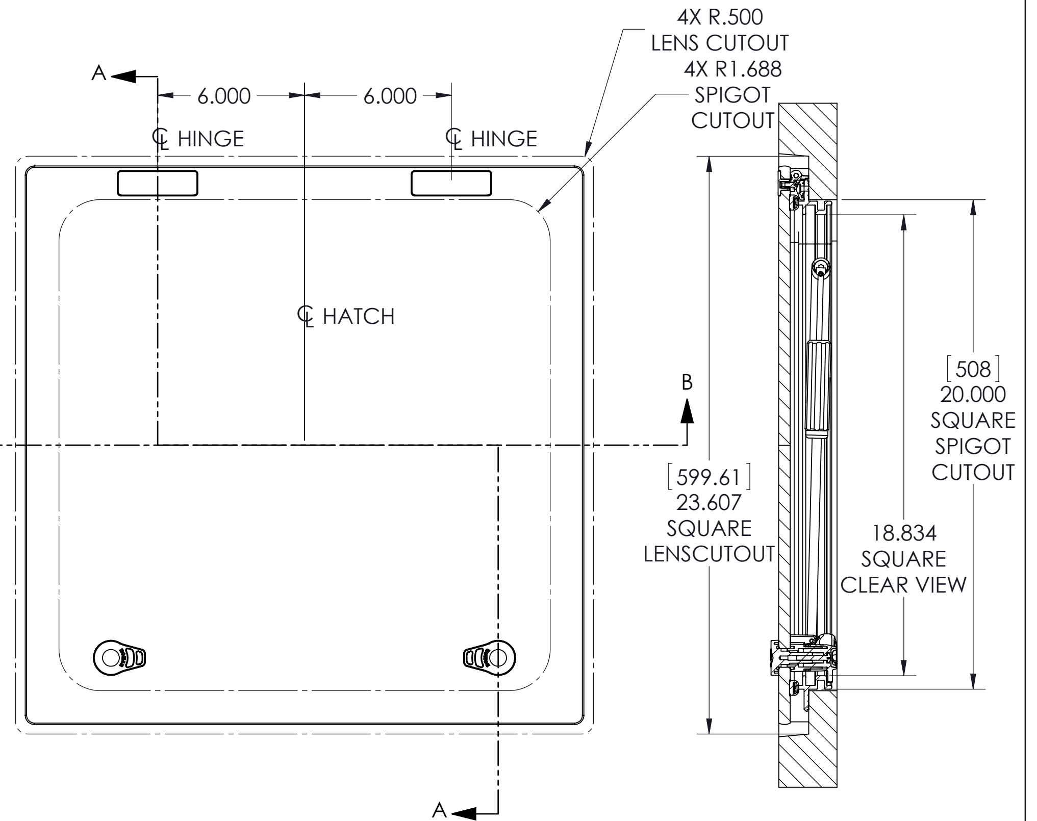
SECTION A-A
